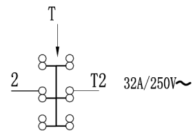
电气图 Electric Diagram: S.P.S.T
